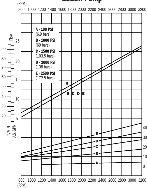
1515K Pump
