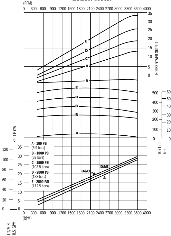
1515K Motor
