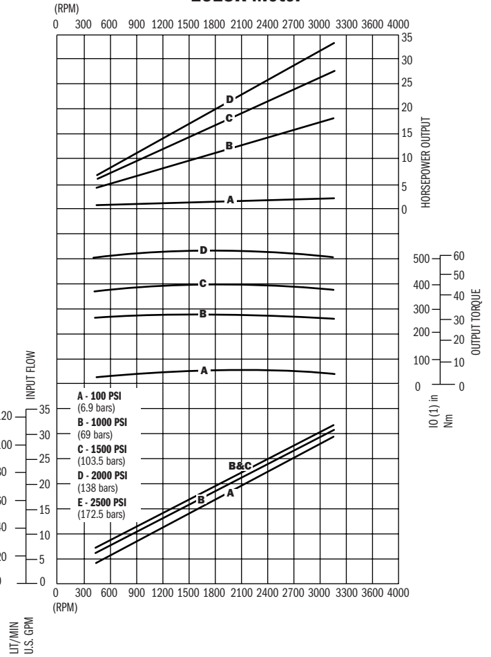
1518K Motor
